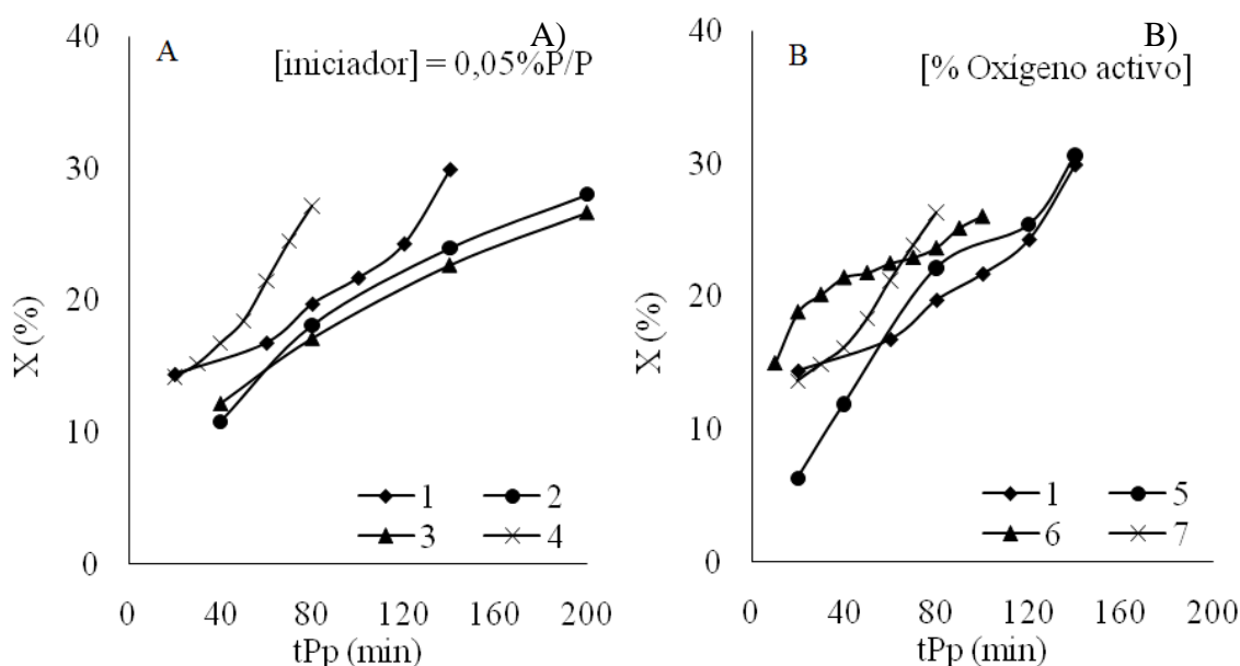
Figura 1. Evolución de la conversión de PS en función del tiempo de pre-polimerización bajo A) la misma concentración de iniciador y B) misma concentración de oxígeno activo.
