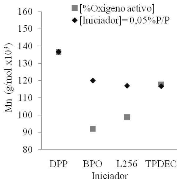
Figura 2. Evolución del peso molecular promedio en número de la matriz de poliestireno de los HIPS, obtenidos bajo la misma concentración de iniciador y misma concentración de oxígeno activo.
